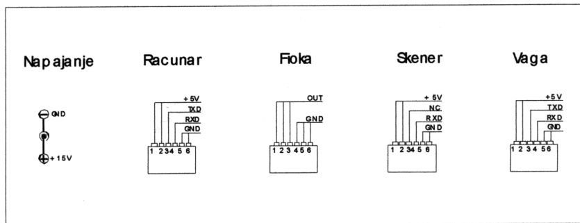
Slika3 - Priklučci kase BINGO PLUS SR
