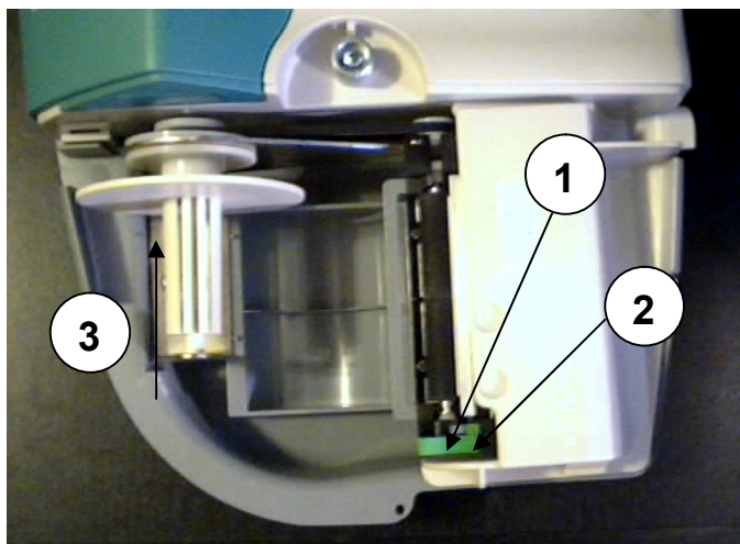
Slika 9 – Mehanizam štampača i element za namotavanje kontrolne trake.
