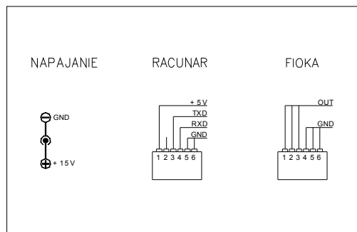
Slika 5 - Priključci kase BINGO STANDARD SR
